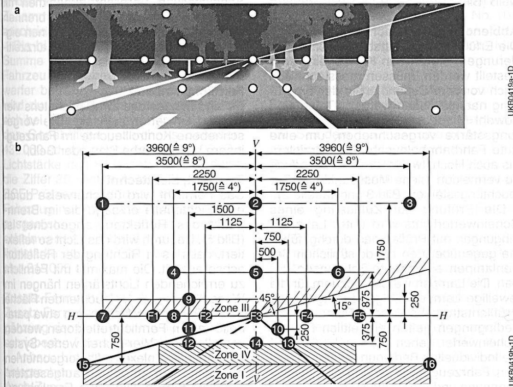
Bild 3: Beleuchtungsstärken der Scheinwerfer für Europa/ECE.
